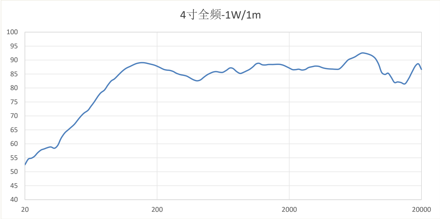
频响曲线
