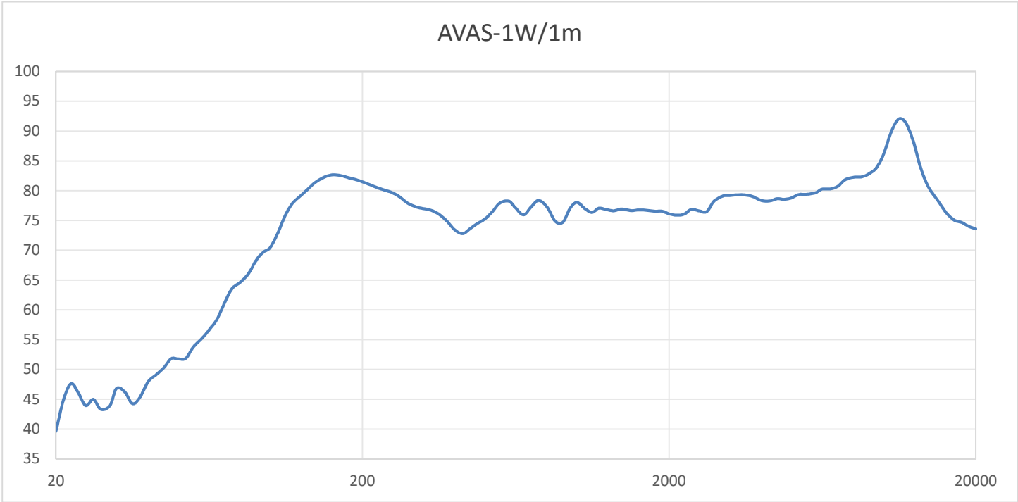
频响曲线
