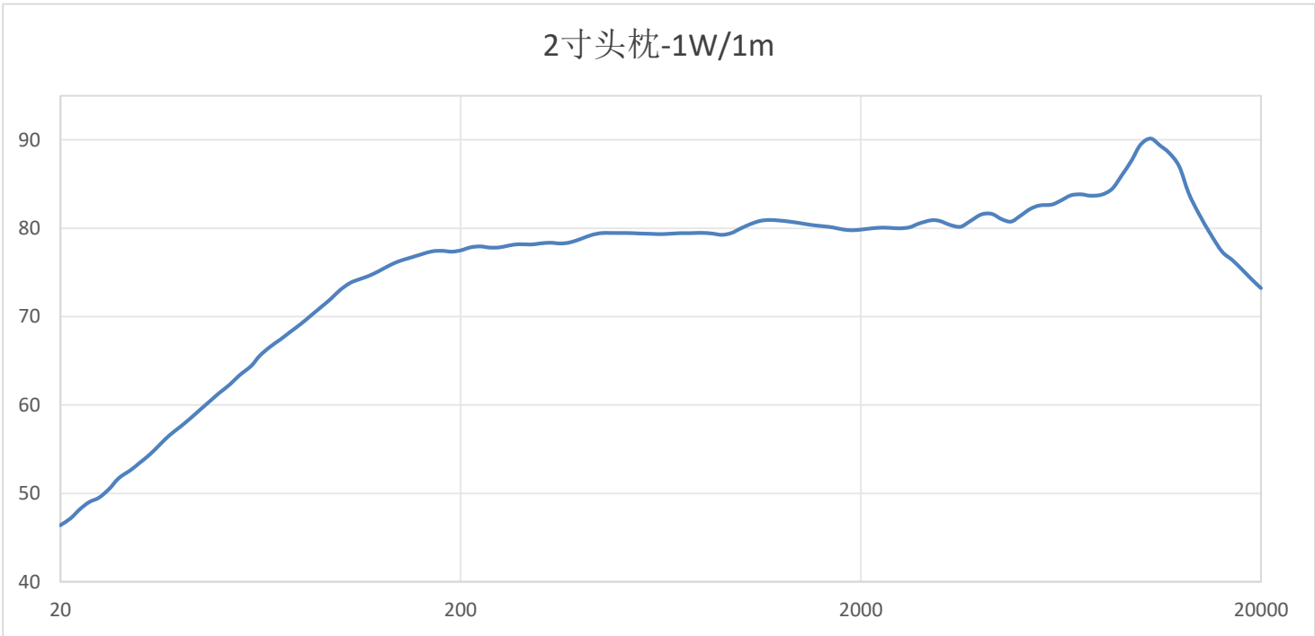
频响曲线
