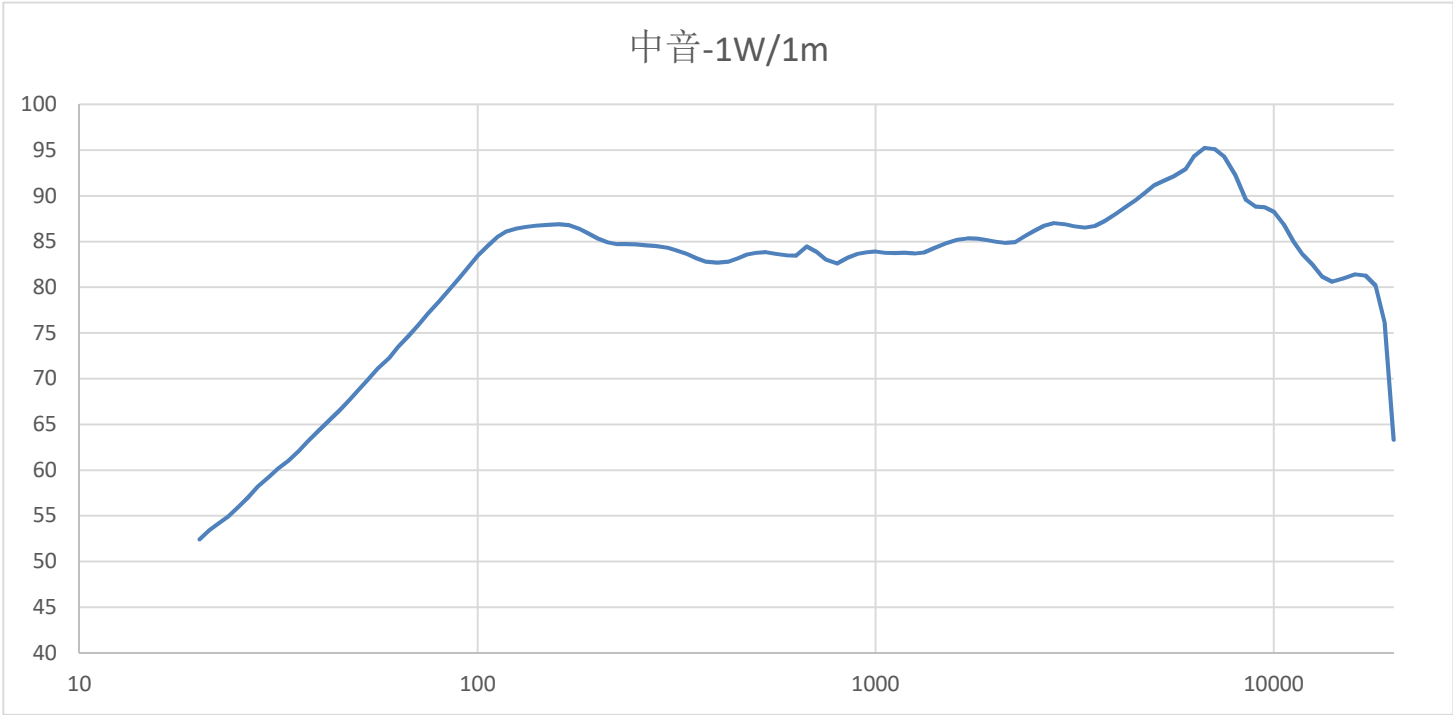
频响曲线
