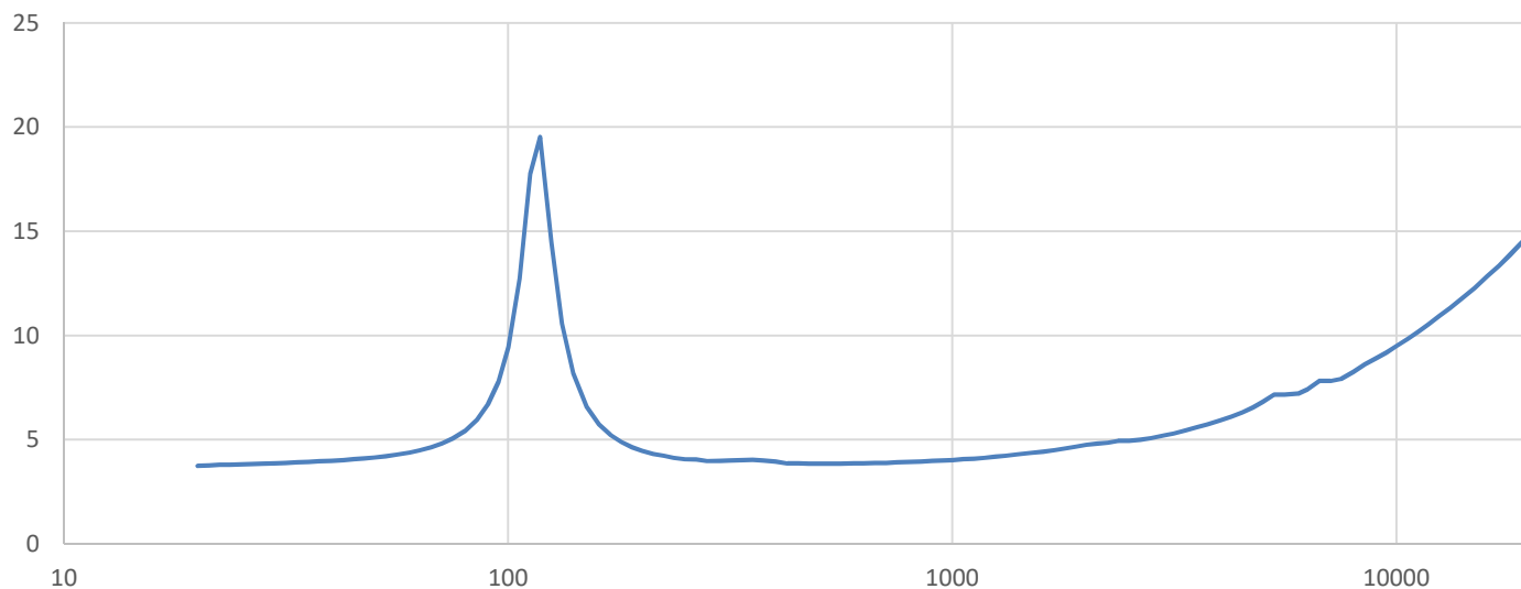
中音-1W/1m
