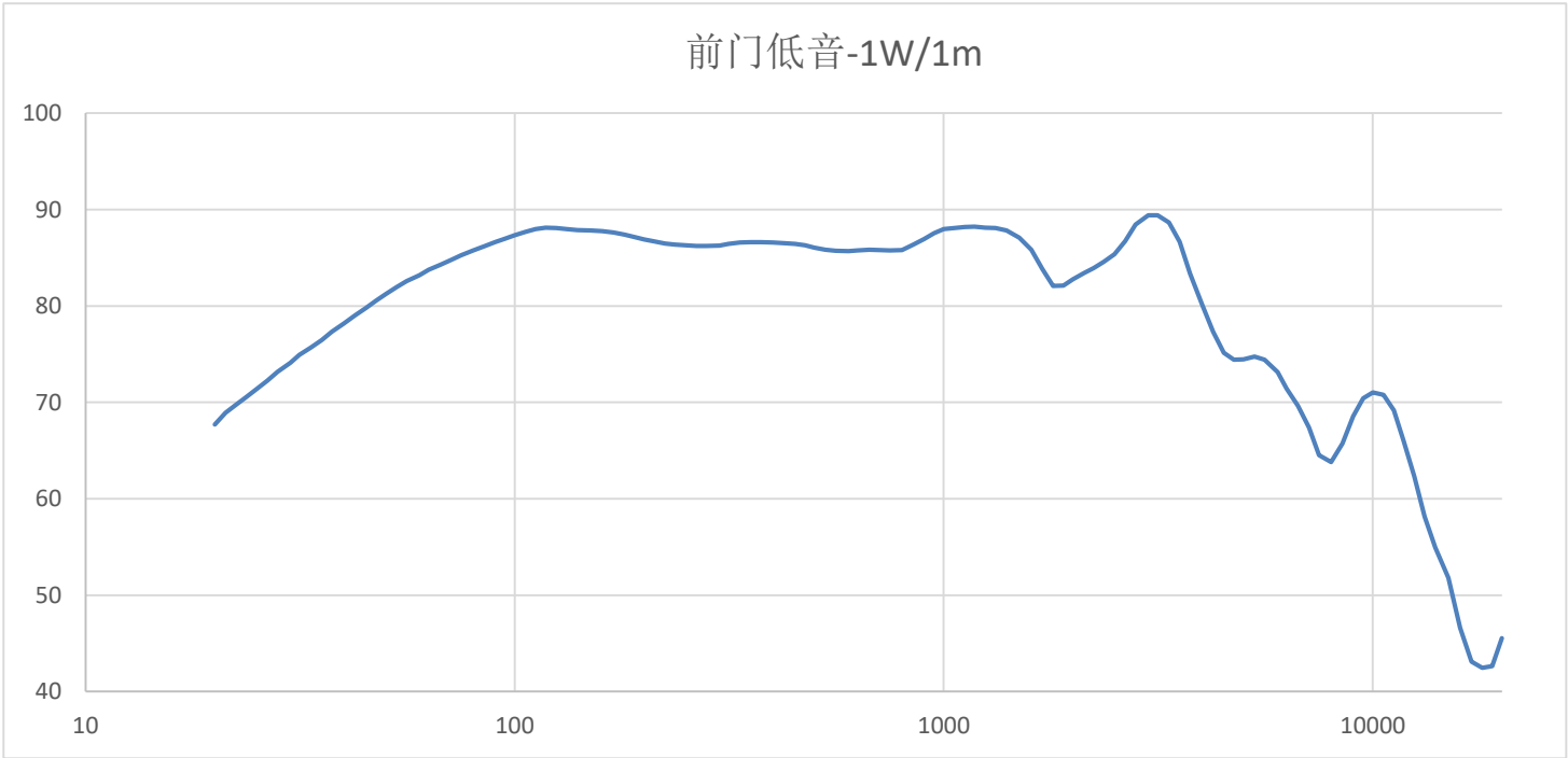
频响曲线
