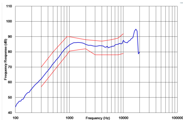
图1 典型频响曲线
