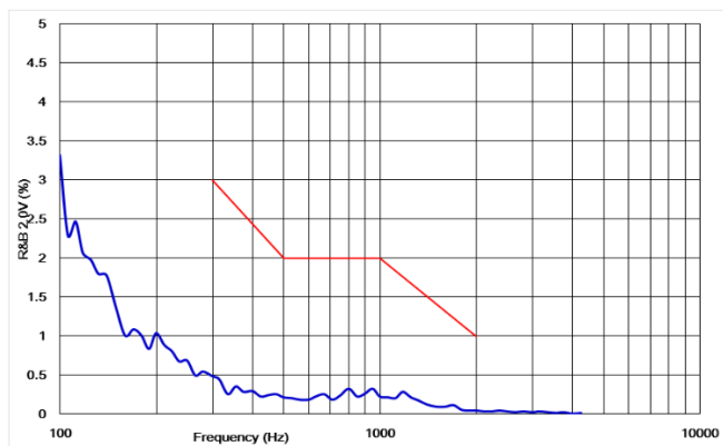
图 3 高次谐波失真曲线
