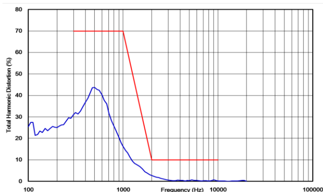
图2 总谐波失真曲线
