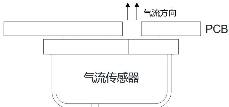
图 4 组装示意图
